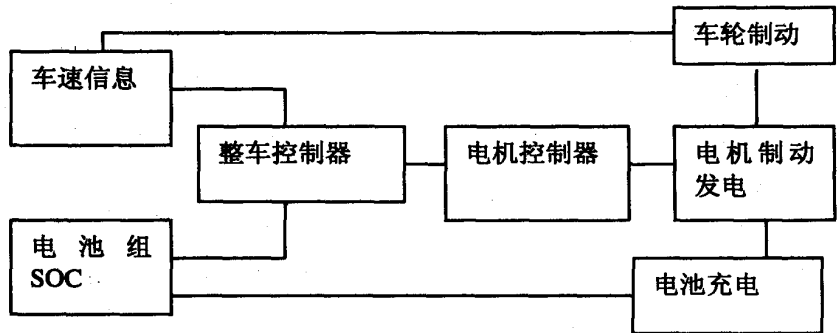
图 2 再生制动功能框图 Fig.2 Function figure of reborn breaking
