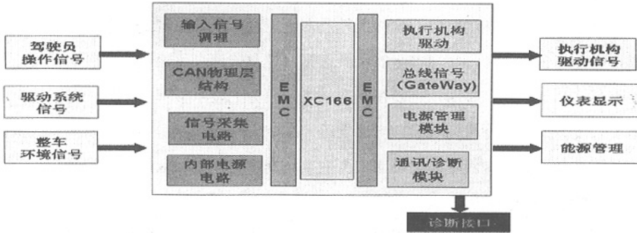
图 7 硬件功能图
